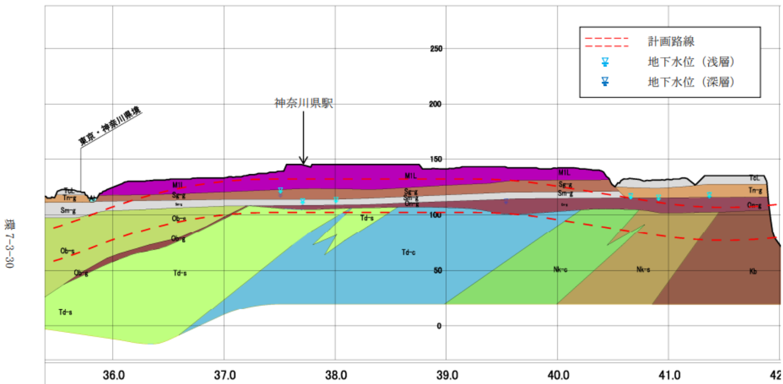
図 7-3-3(4) 都市トンネル区間縦断面図 (相模原地区)
